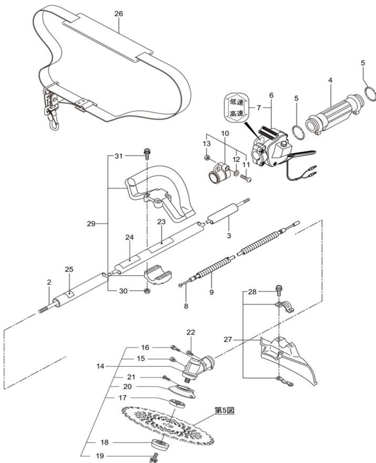
第4図 アタッチメント部
