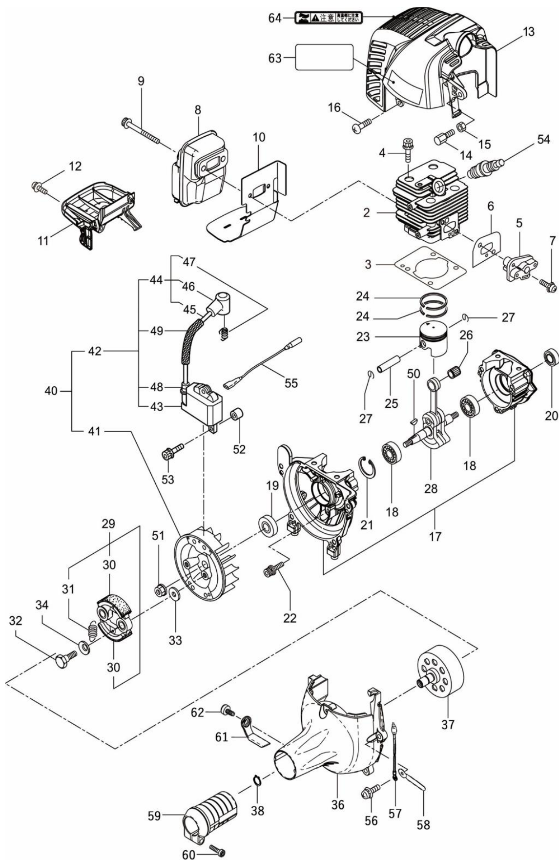
第1図 シリンダー、ピストン、エンジンカバー部
