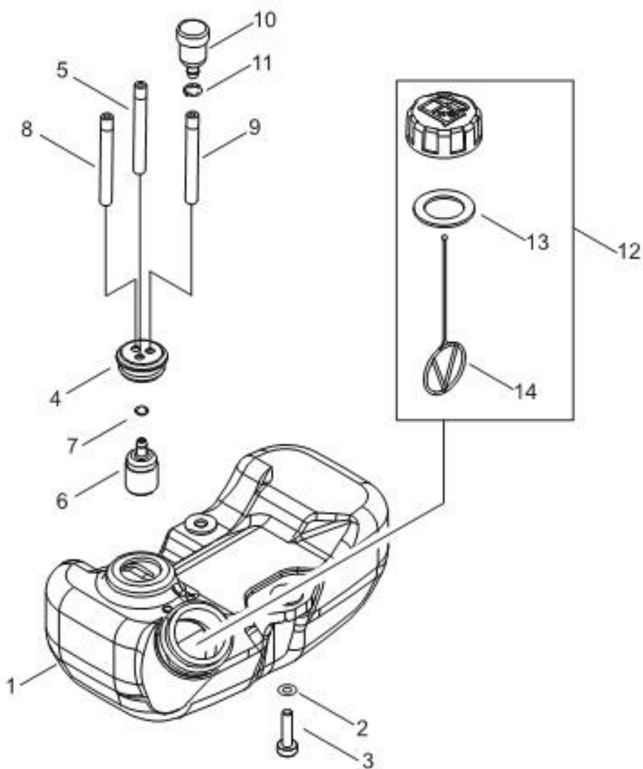
第6図 燃料タンク部
