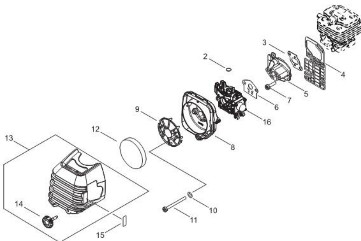
第5図 エアクリーナー・キャブレター部
