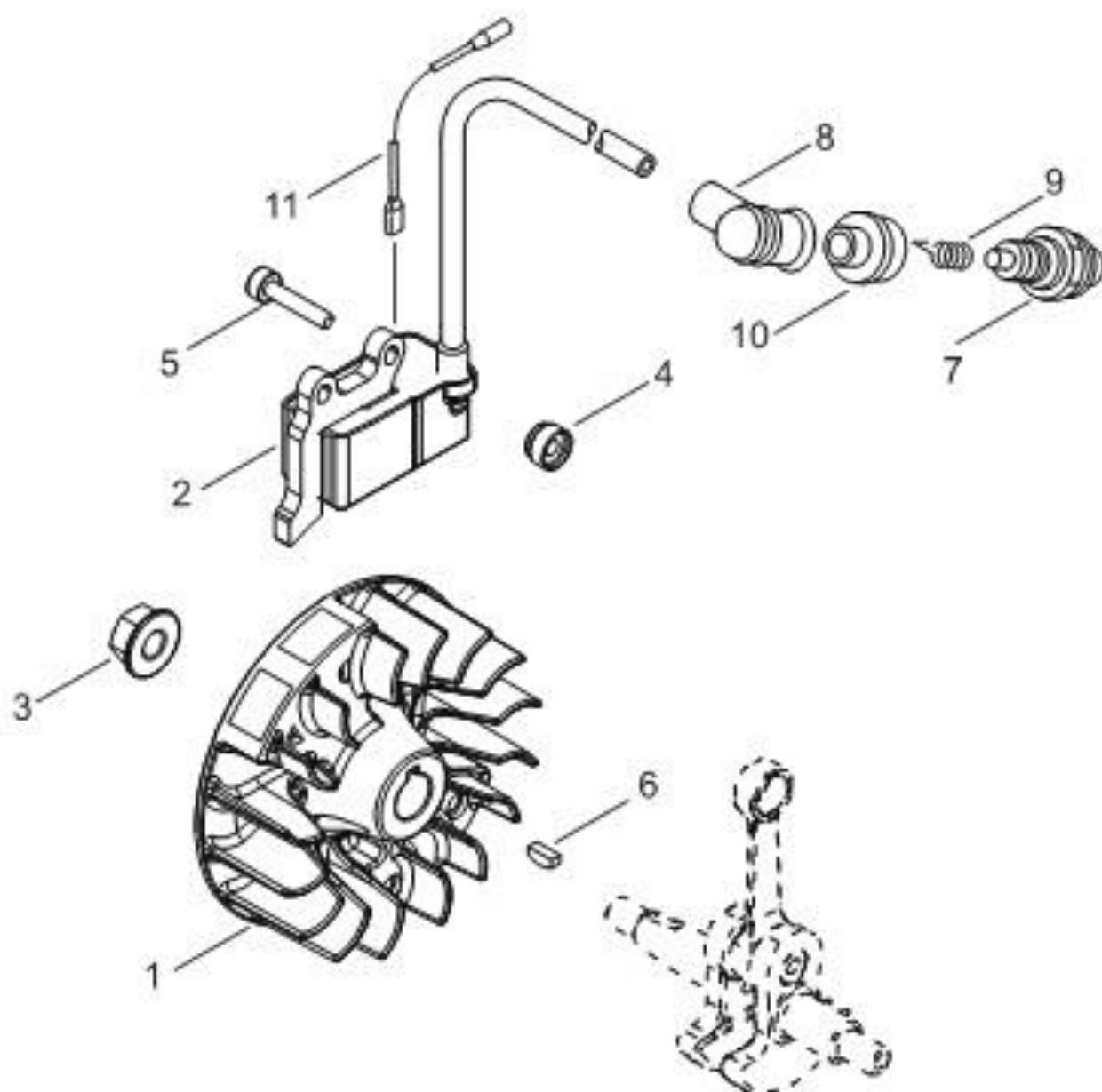
第3図 電装品部
