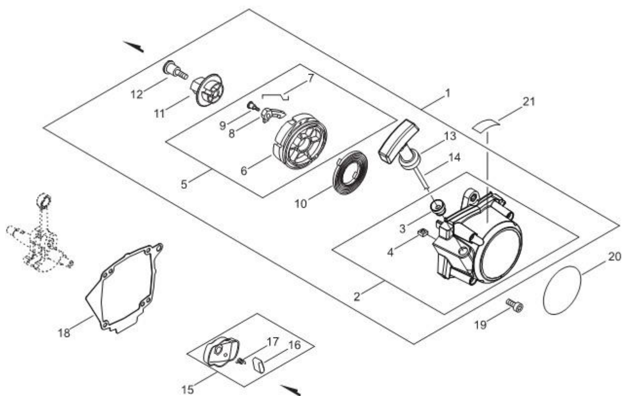
第8図 リコイルスターター部
