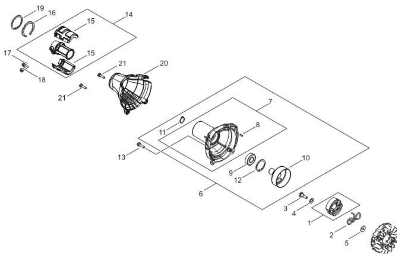
第4図 クラッチ部
