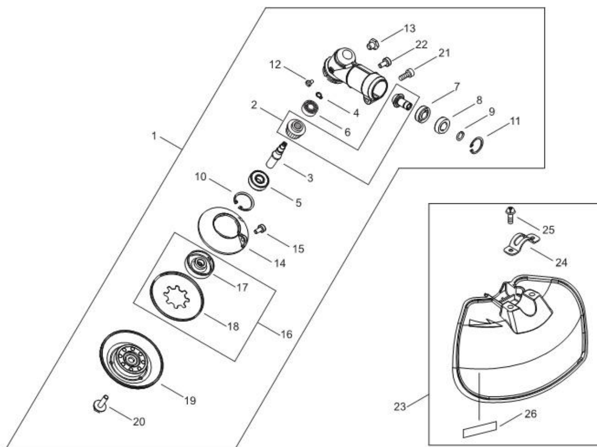
第9図 ギアケース・飛散防護カバー部
