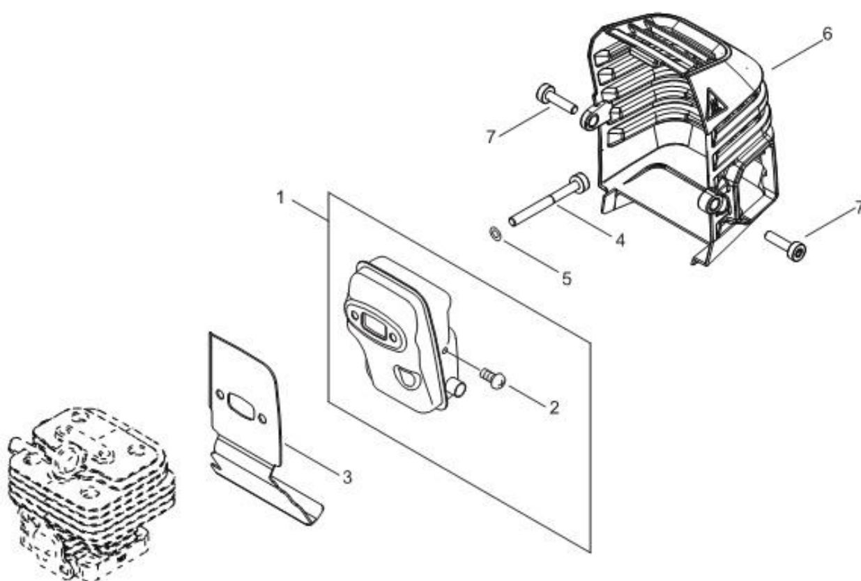
第7図 マフラー部
