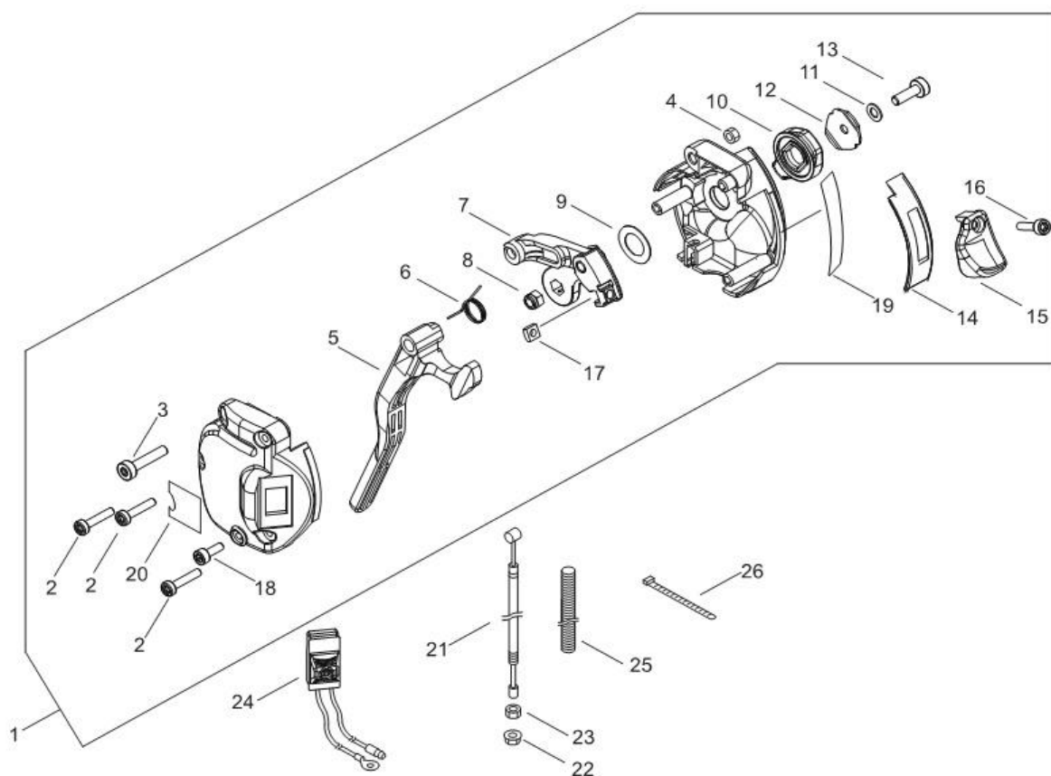
第11図 スロットルレバー部
