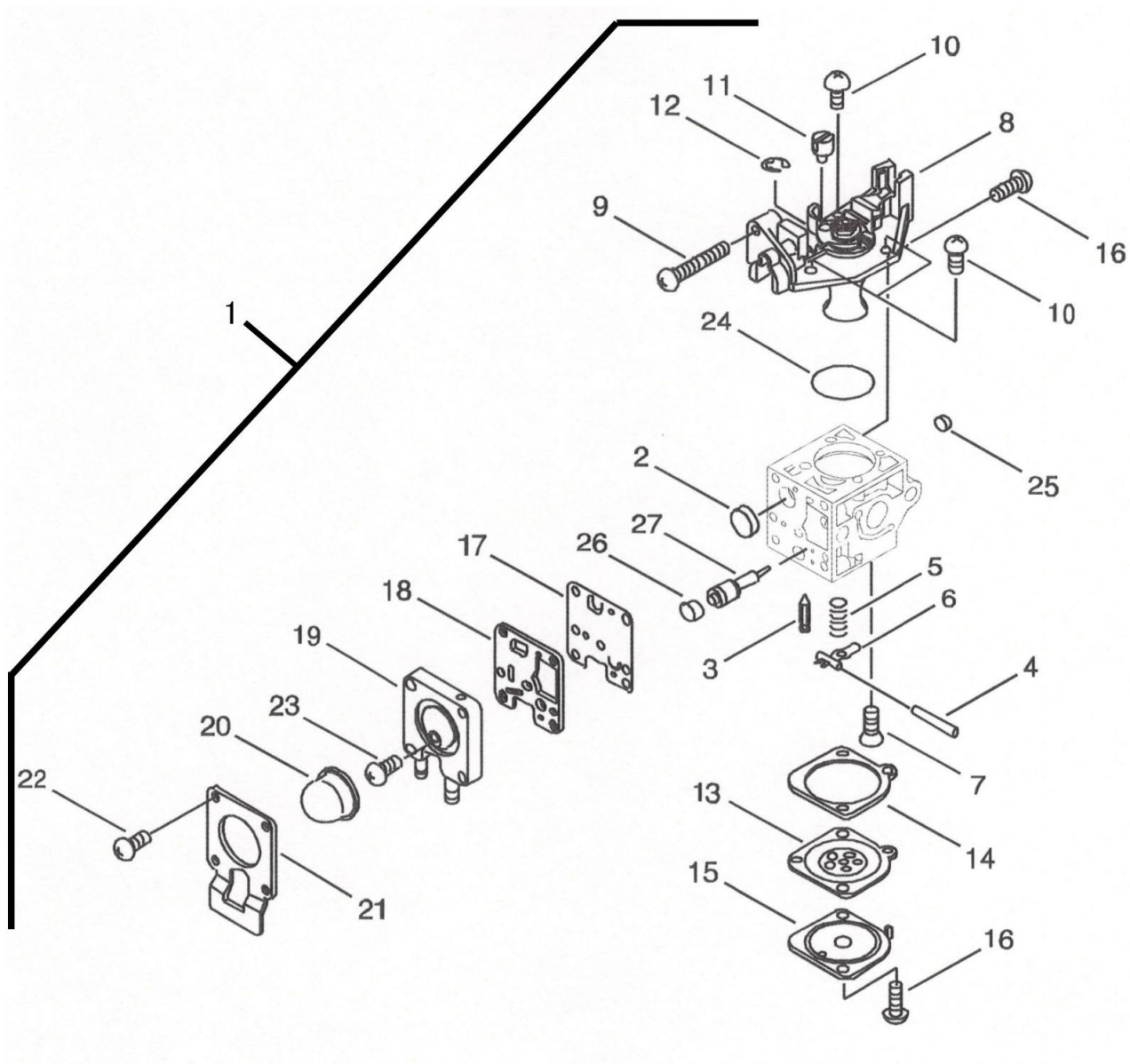
第7図 キャブレター部(シリアル 58101001以前)
