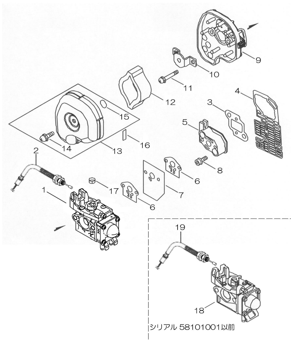
第5図 エアクリーナー部
