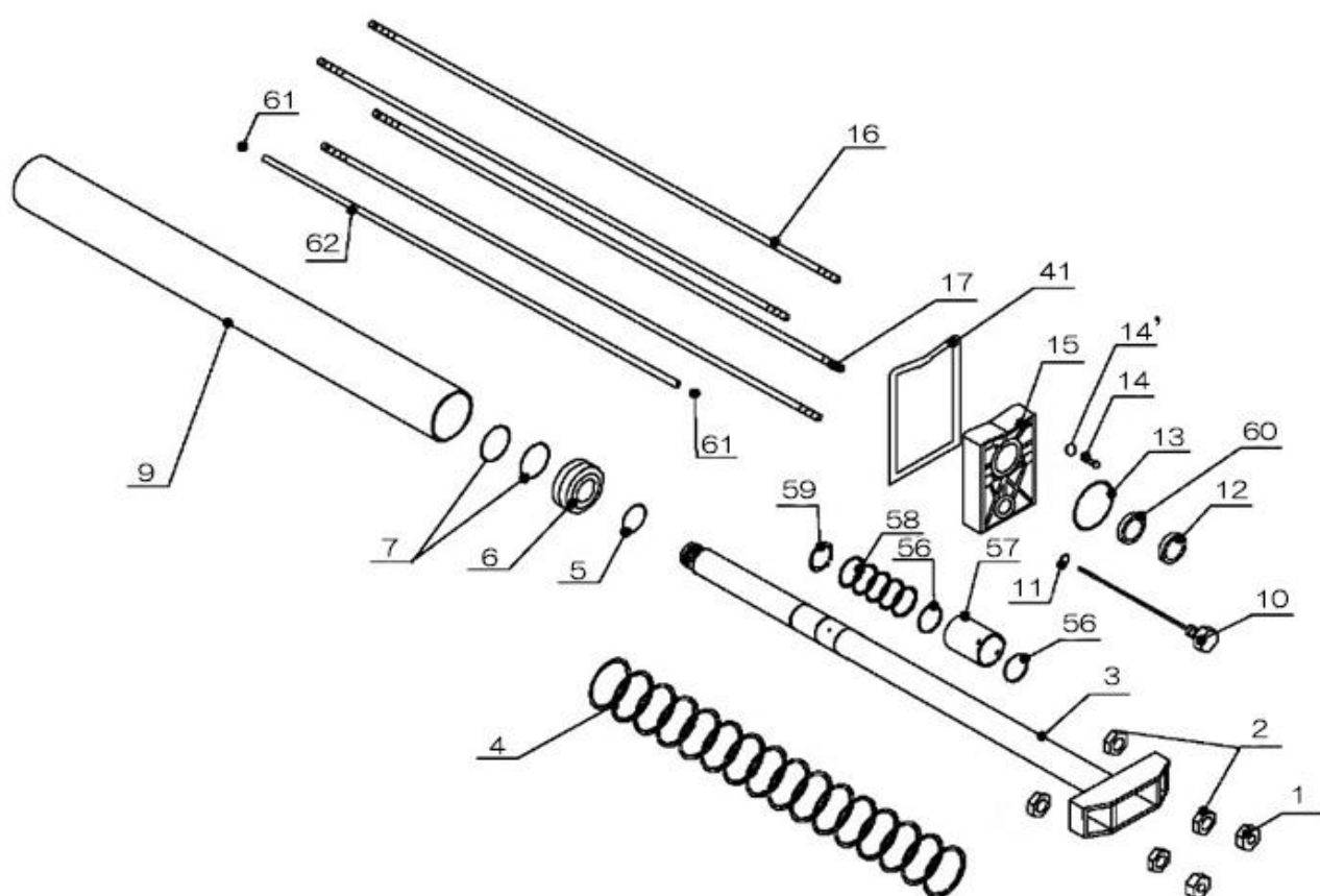
第4図 シリンダー部
