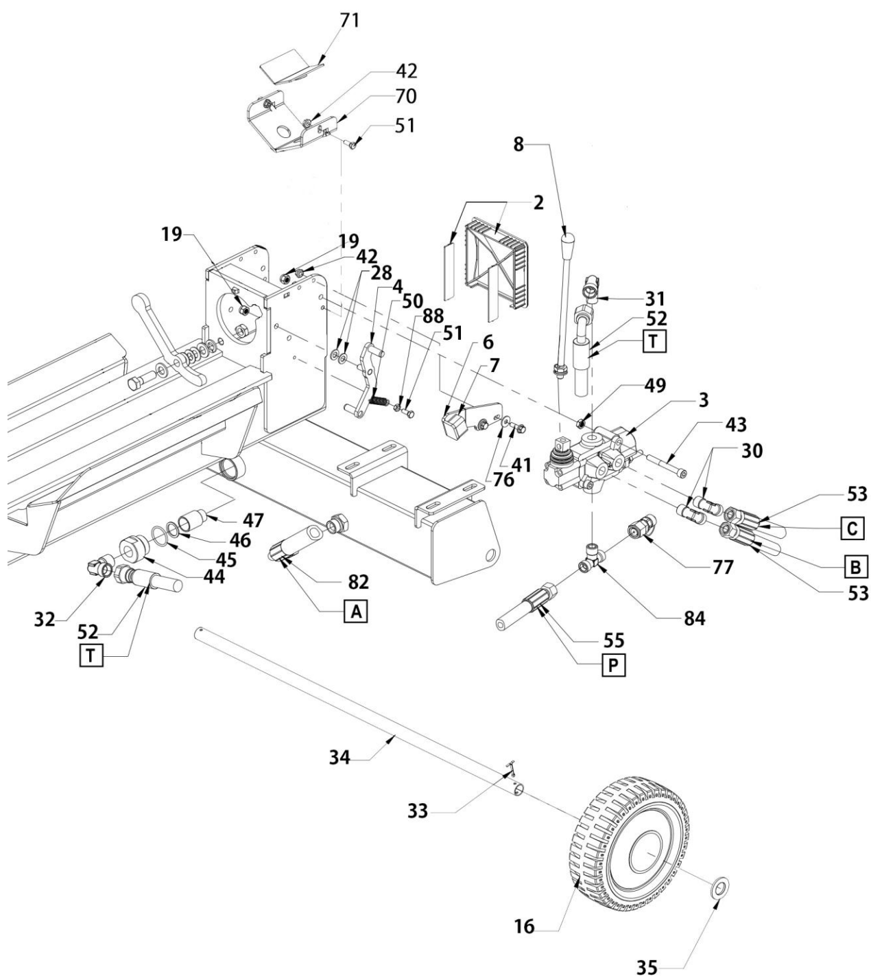
第1図 コントロールバルブ部
