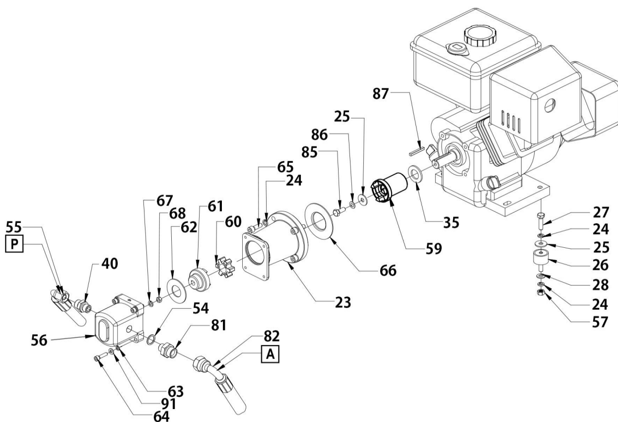
第5図 ポンプ・カップリング・マウント部
