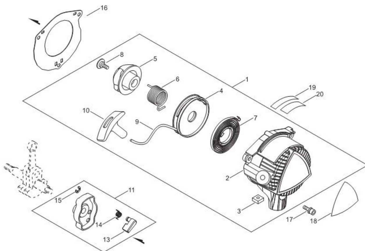
第8図 リコイルスターター部
