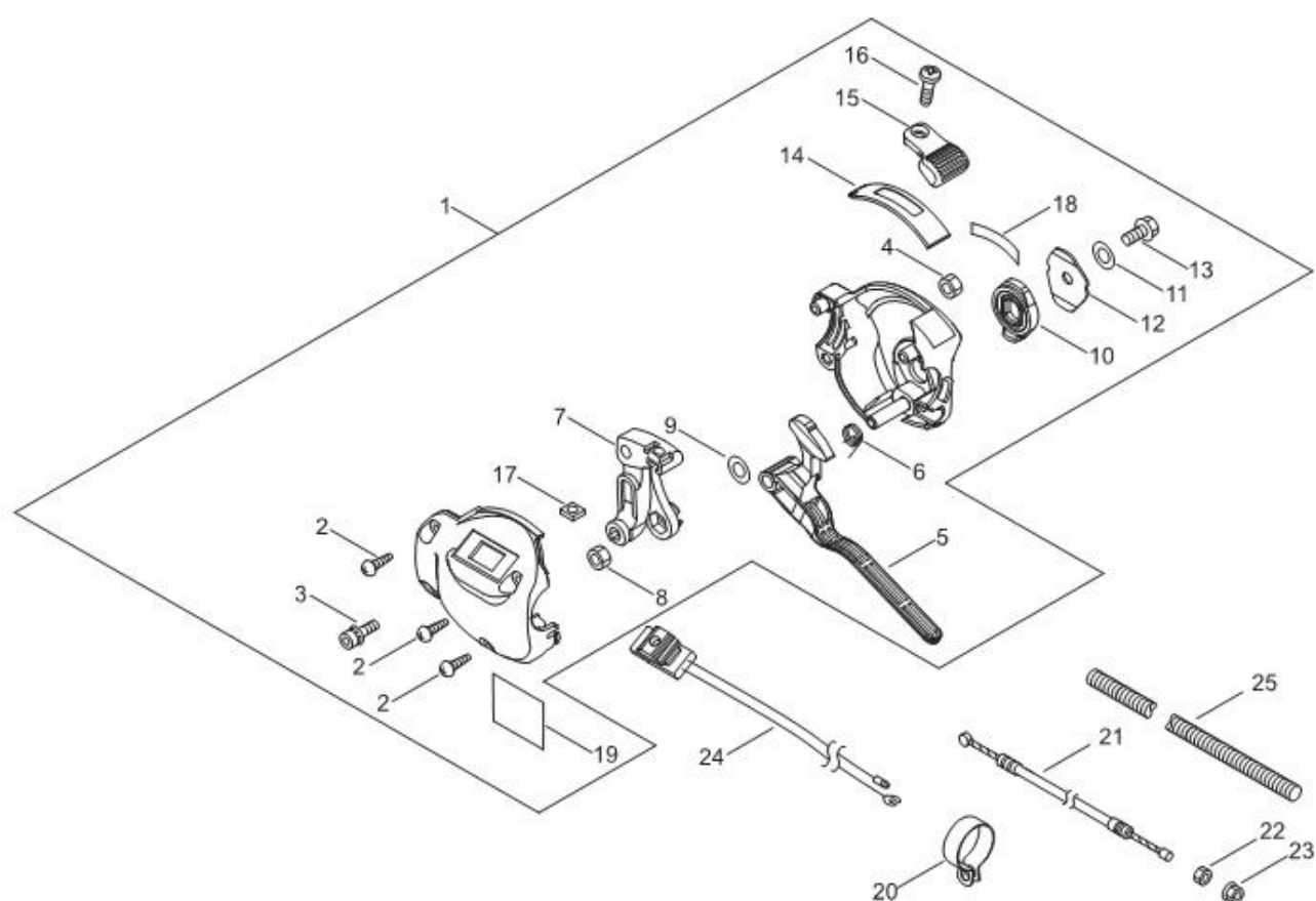
第11図 スロットルレバー部
