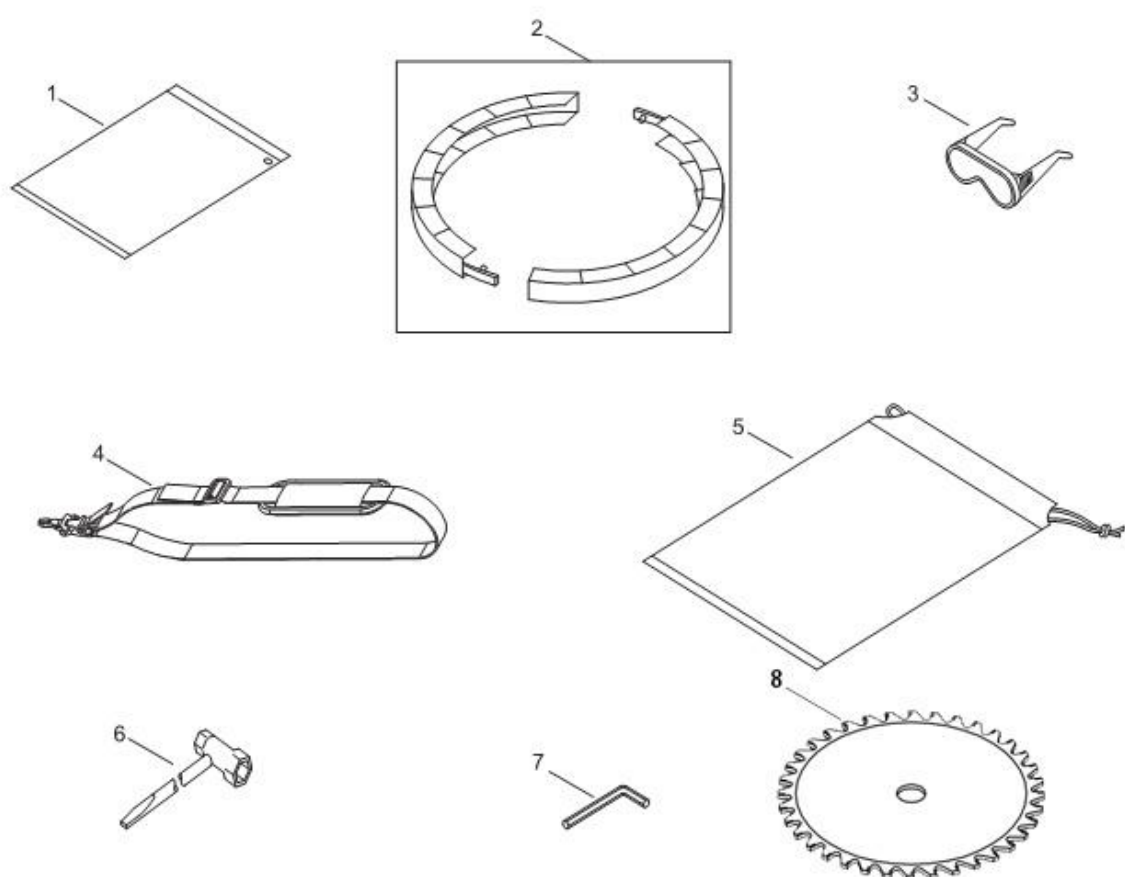
第12図 入組品部
