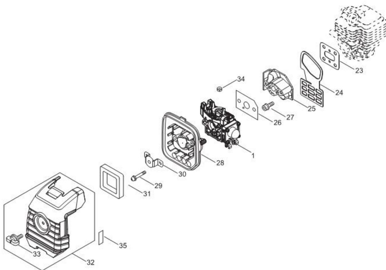
第5図 エアクリーナー・キャブレター部
