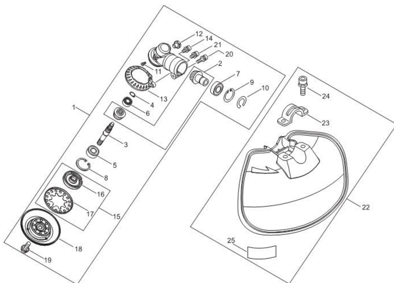
第9図 ギアケース・飛散防護カバー部
