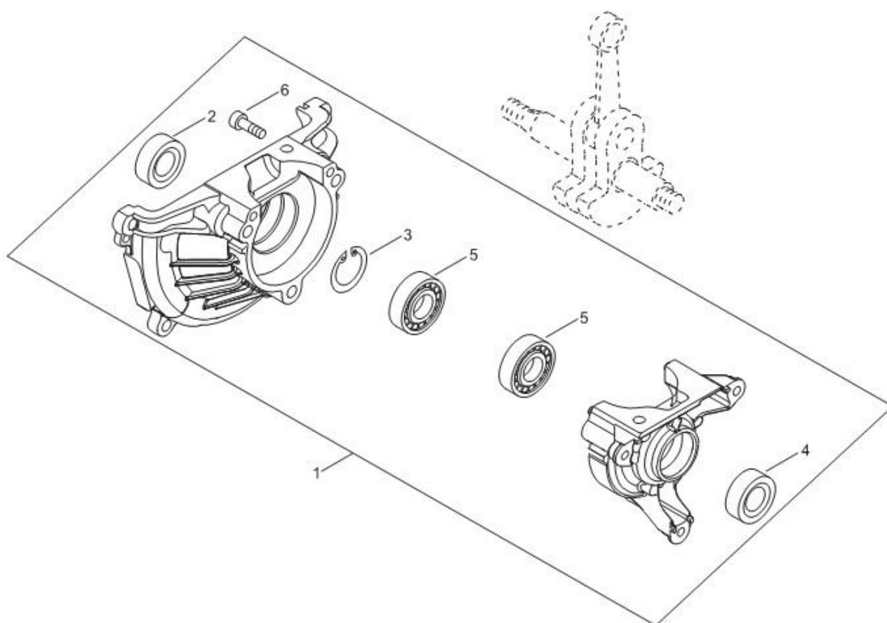
第2図 クランクケース部
