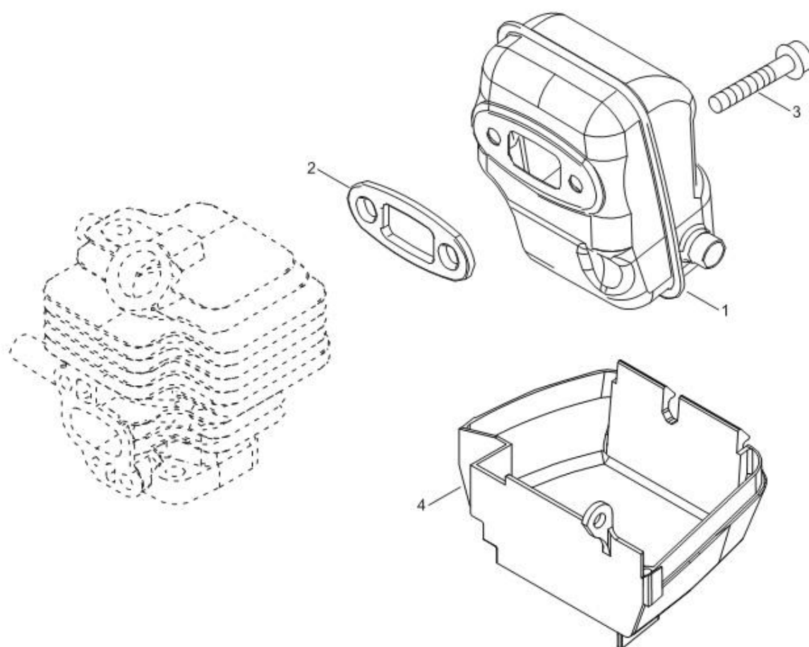
第7図 マフラー部
