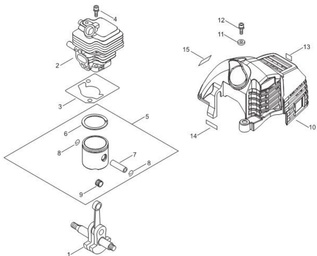
第1図 シリンダー、ピストン、エンジンカバー部
