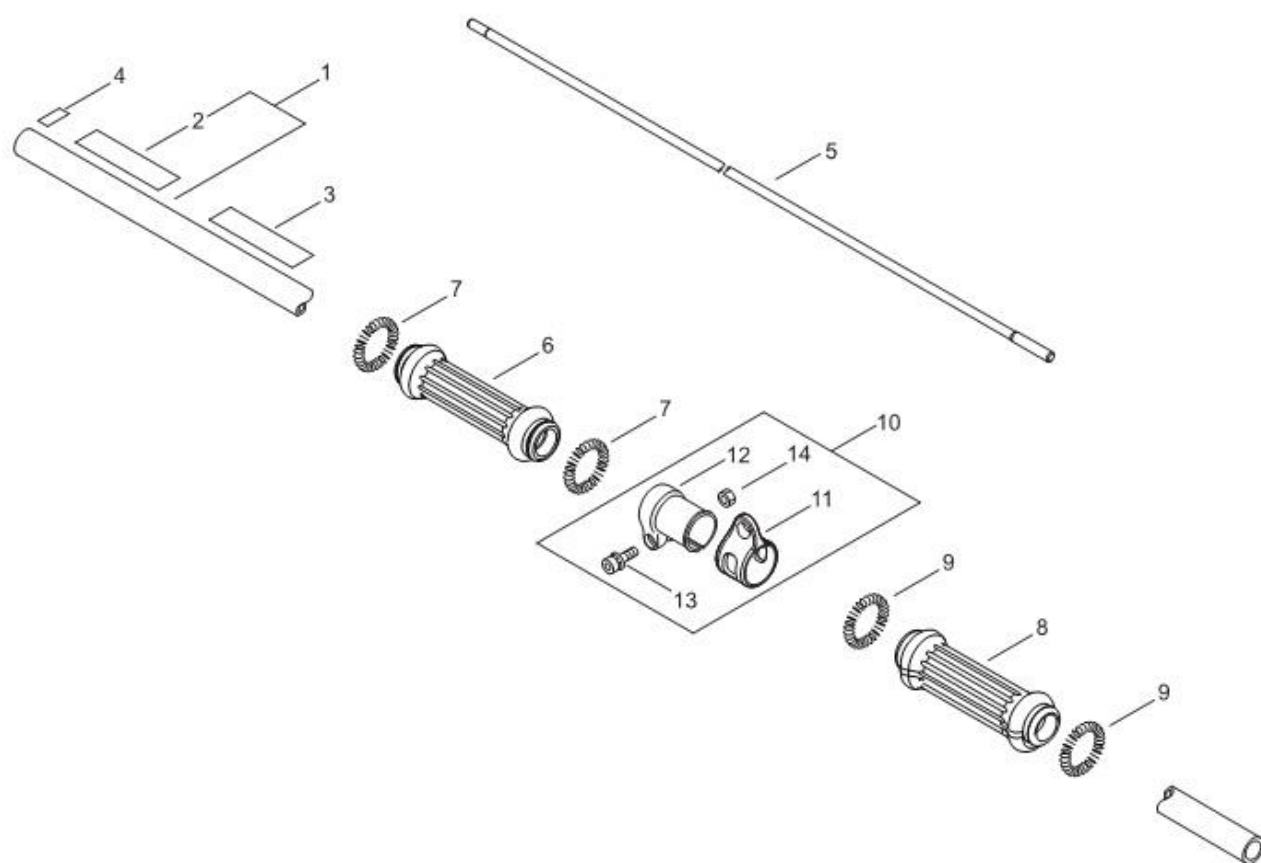
第10図 アタッチメント部
