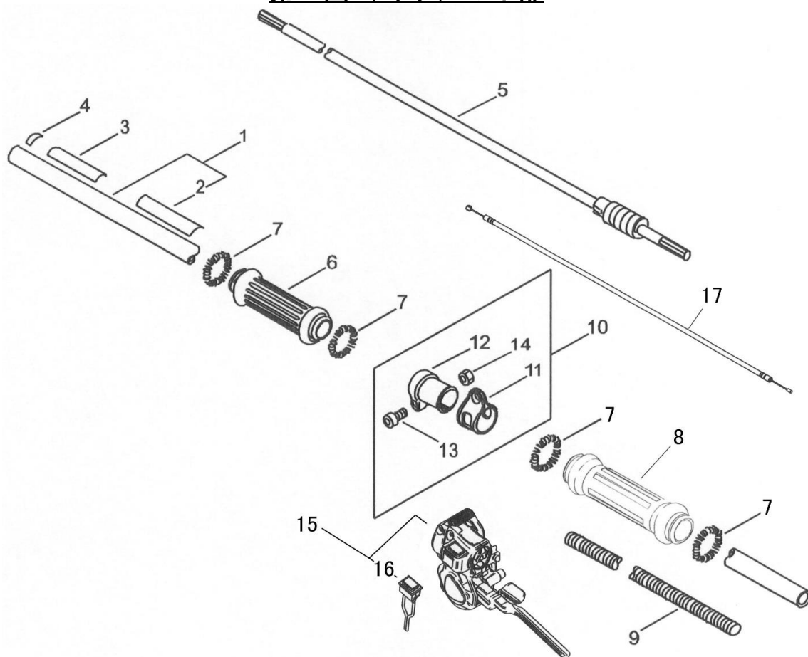
第11図 アタッチメント部
