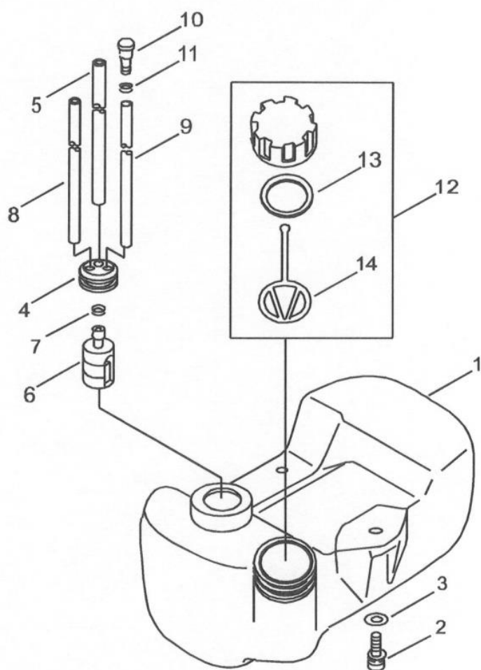
第6図 燃料タンク部
