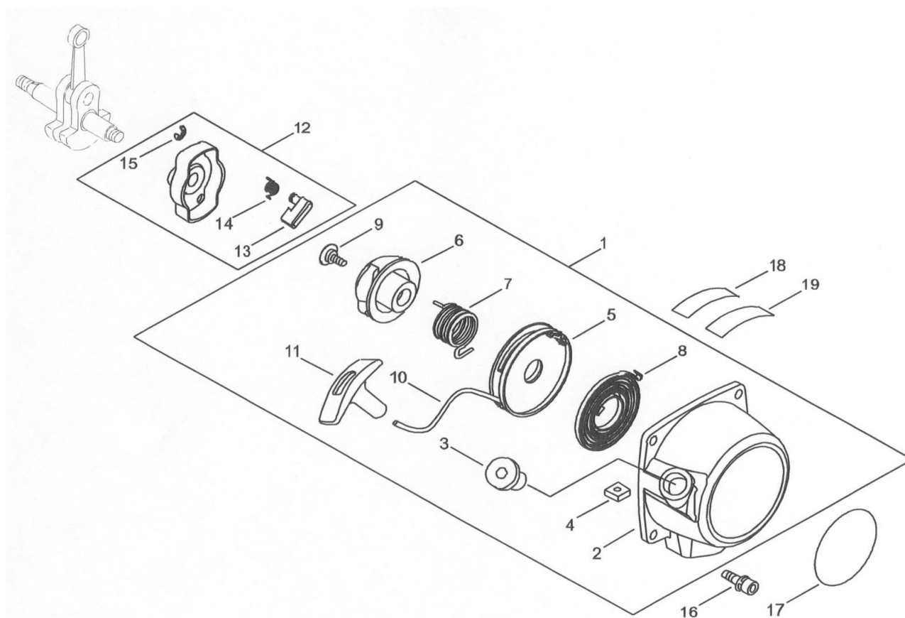
第9図 スターター一部
