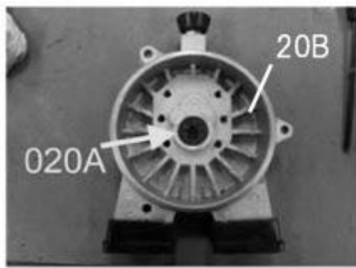
第2図 ポンプ、モーター部
